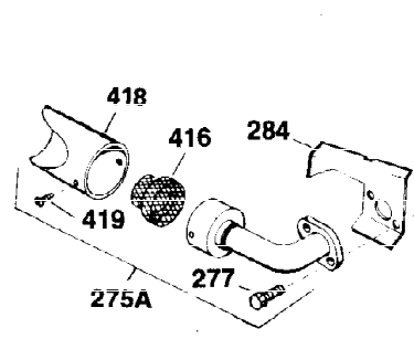
OPTIONAL SPARK ARREST MUFFLER
